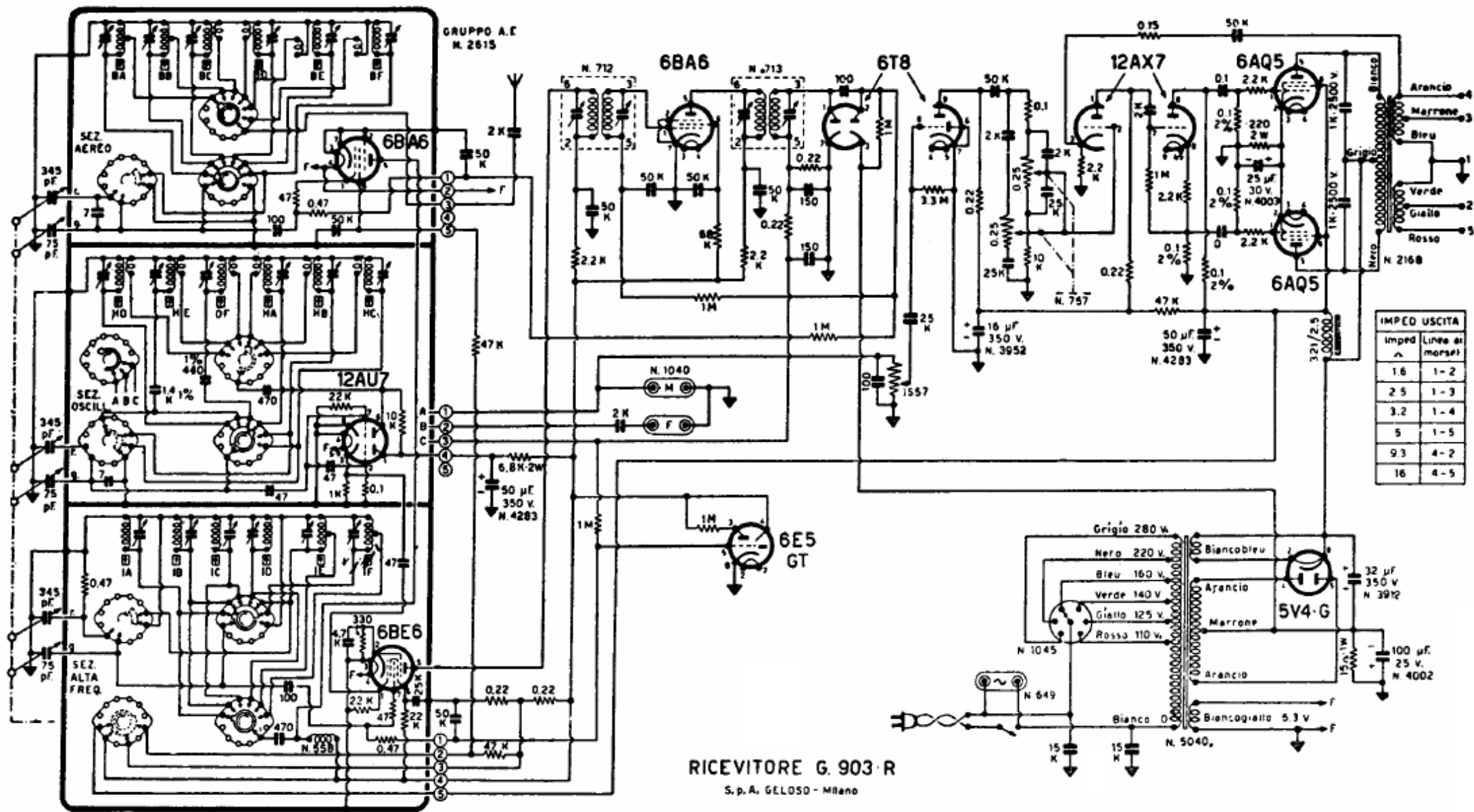
GELOSO - Mod. G.903-R. Onde medie e cinque gamme onde corte. Amplificazione finale in controfase, con potenza d'uscita da 8 a 11 watt. Sensibilità d'antenna 2 \mu\text{V} per 60 mw d'uscita. MF a 467 kc/s. Controlli alti e bassi.
